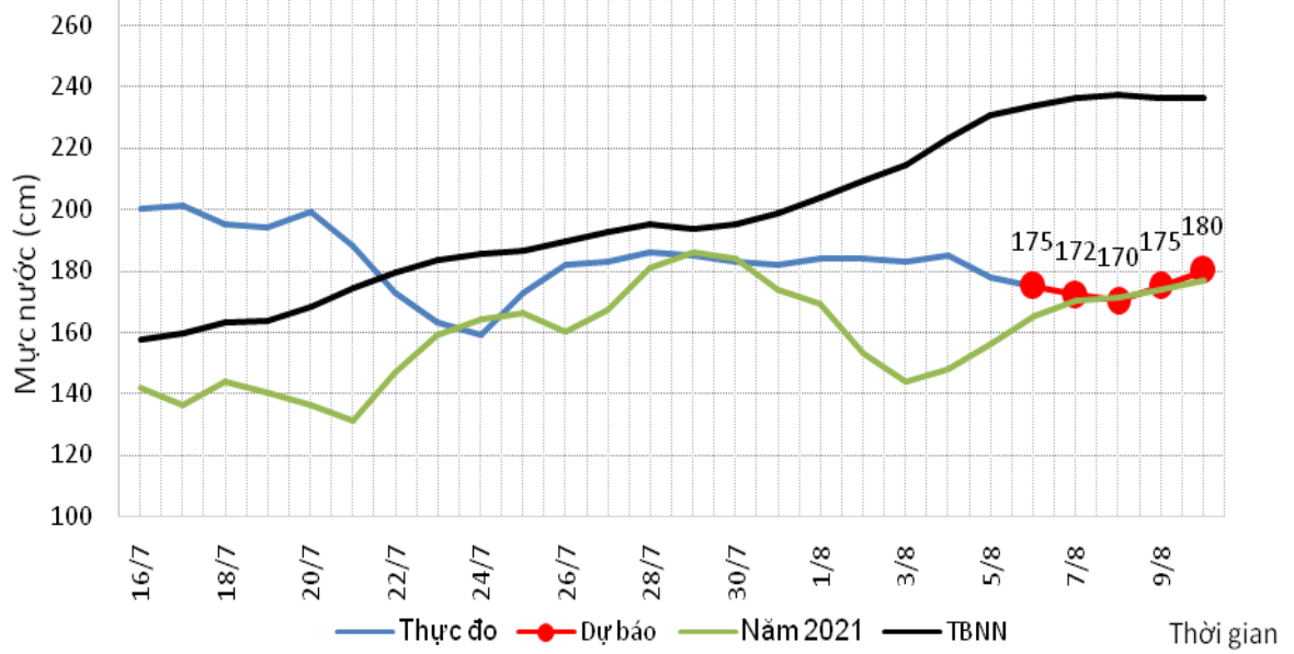
QUÁ TRÌNH MỨC NƯỚC THỰC ĐO VÀ DỰ BÁO TRẠM TÂN CHÂU (SÔNG TIỀN)
